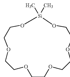
dimethylsila-17-crown-6.
